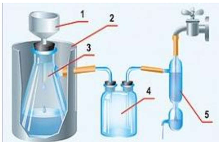
სურათი 4. 97. ვაკუუმ-ფილტრაციის მოწყობილობა. 1. ბიუნზერის ძაბრი; 2. დამცავი გარსაცმი; 3. ბუნზენის კოლბა; 4. დამცავი ჭურჭელი; 5. წყალჭავლური ტუმბო
