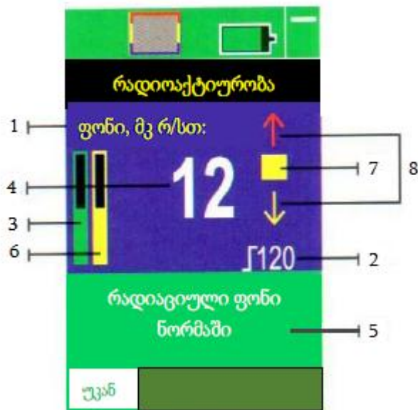
სურათი 2.26. ეკოტესტერი „SOEKS“-ის მენიუ
