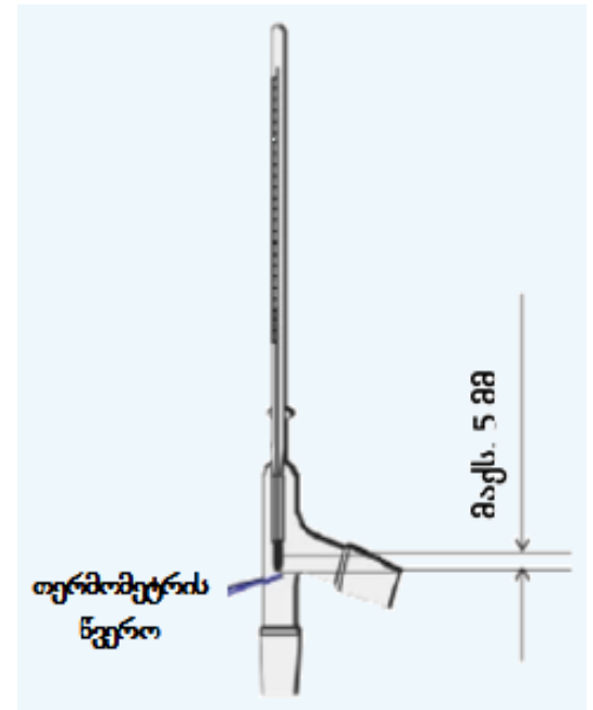
სურათი 4. 98. თერმომეტრის მორგება კოლბაზე
