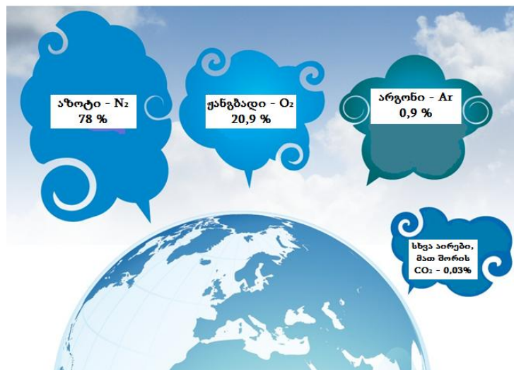
სურათი 1.5. ატმოსფერული ჰაერის შემადგენლობა
