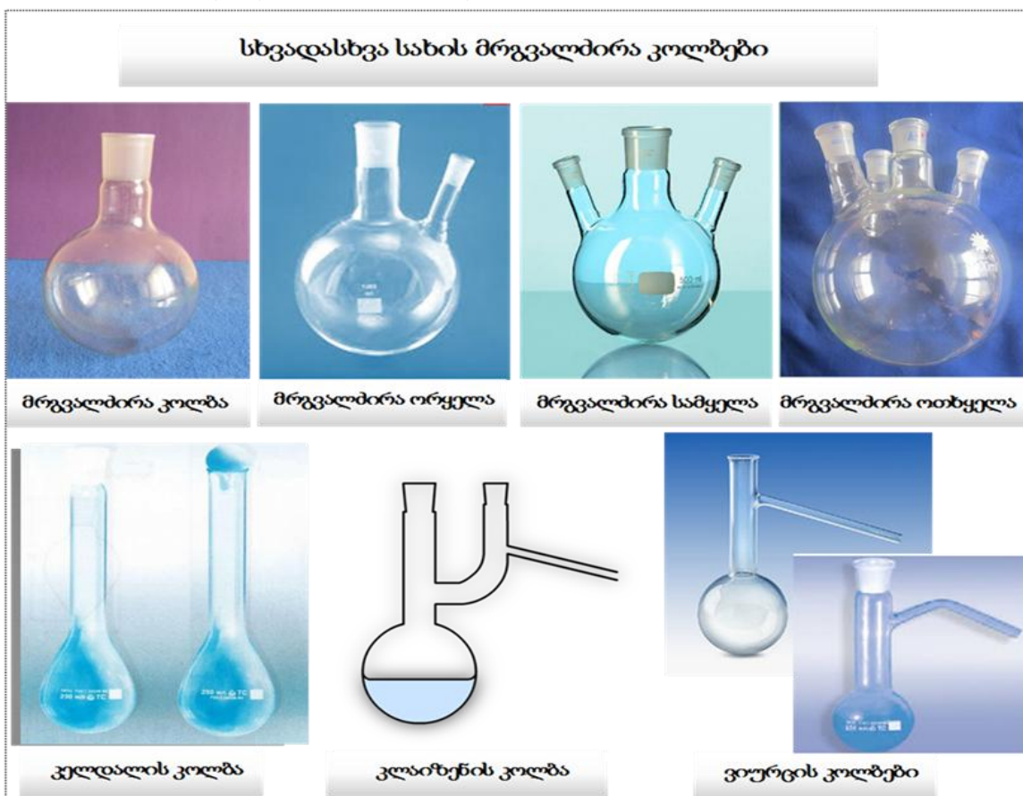
სურათი 4.14. მრგვალძირა კოლბები
