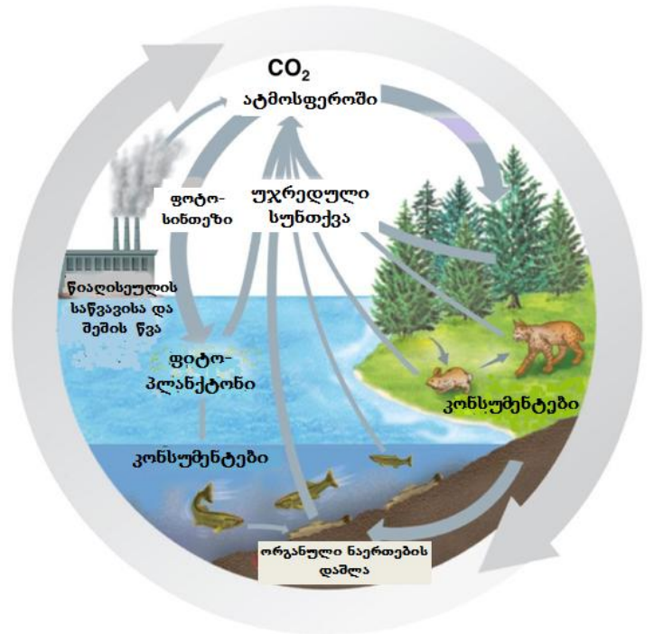
სურათი 1.8. ნახშირბადის წრებრუნვა (გამარტივებული სქემა)
