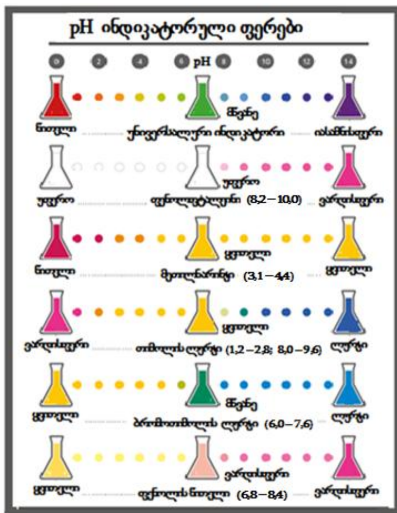
სურათი 4. 88. ინდიკატორების ფერის გადასვლა სხვადასხვა pH-ის დროს
