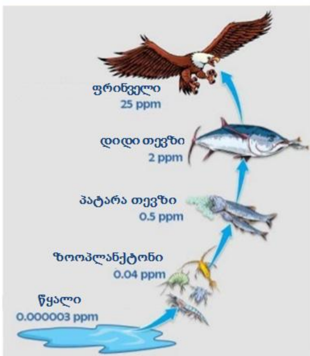
სურათი 1.18. დღტ-ს ბიომაგნიფიკაცია და ბიოაკუმულაცია
