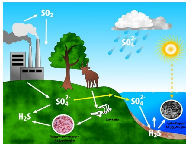
სურათი 1.13. გოგირდის წრებრუნვა
