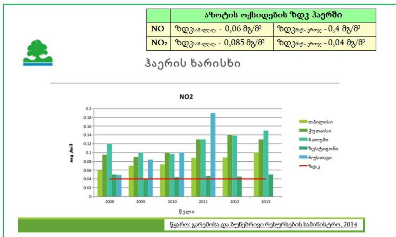
სურათი 2.10. \text{NO}_2 -ის კონცენტრაცია ჰაერში, საქართველო, 2008-2013 წ
