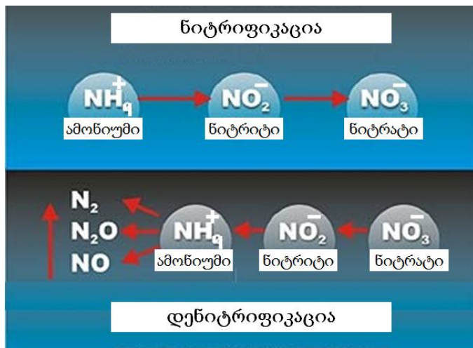
სურათი 1.11. ნიტრიფიკაციისა და დენიტრიფიკაციის პროცესი
